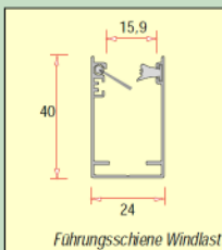
Führungsschiene Windlast
